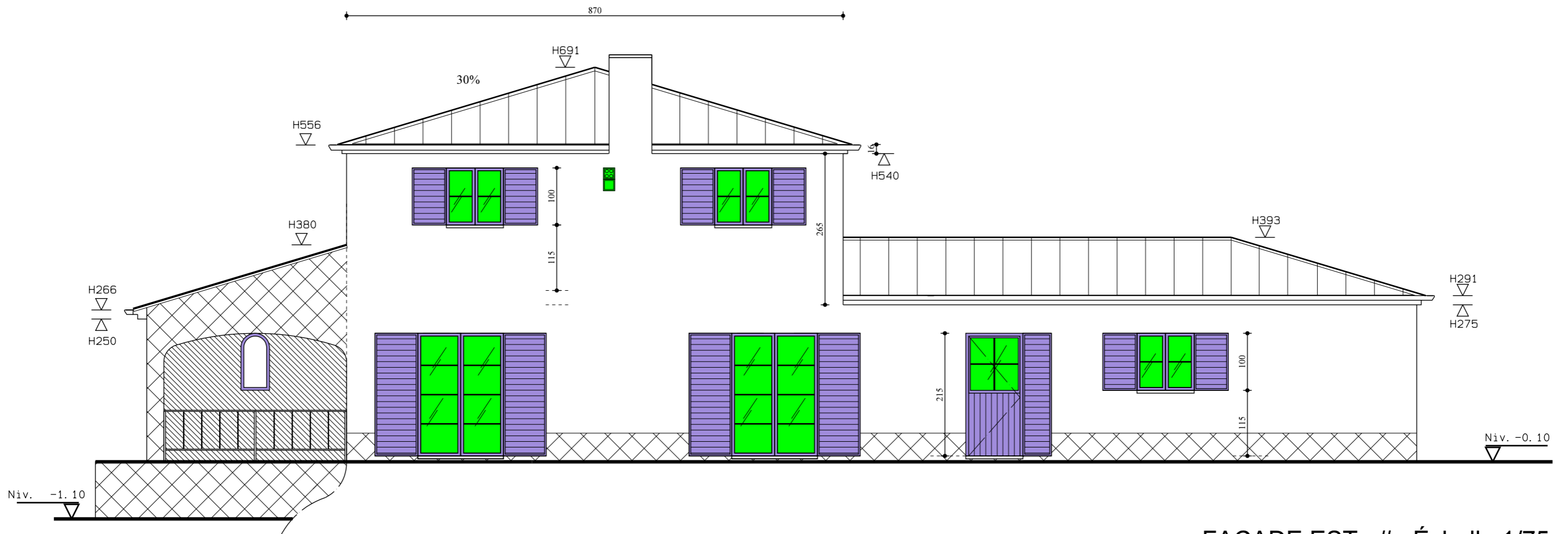
FACADE EST # Échelle 1/75
